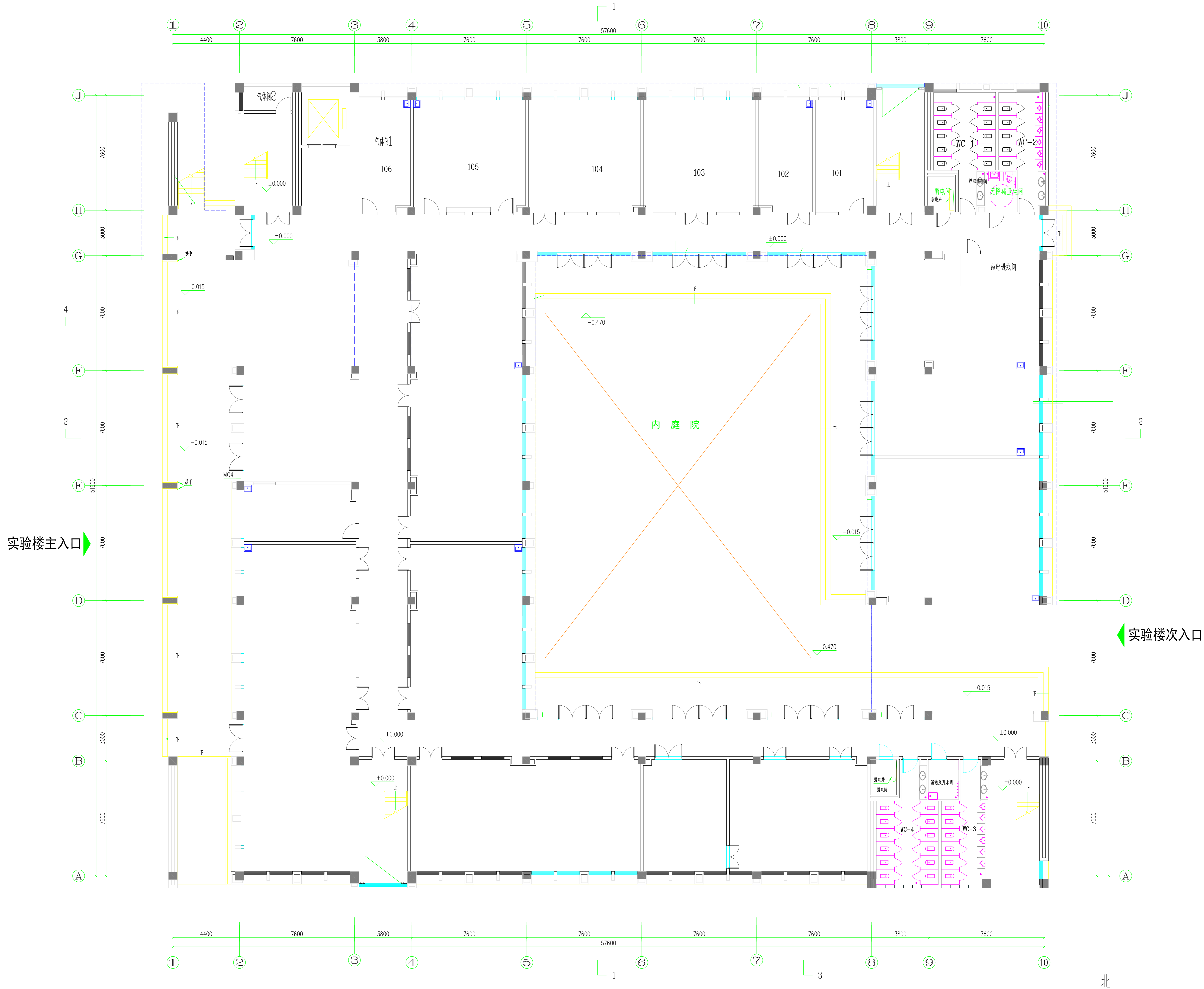
首层平面 1:100
