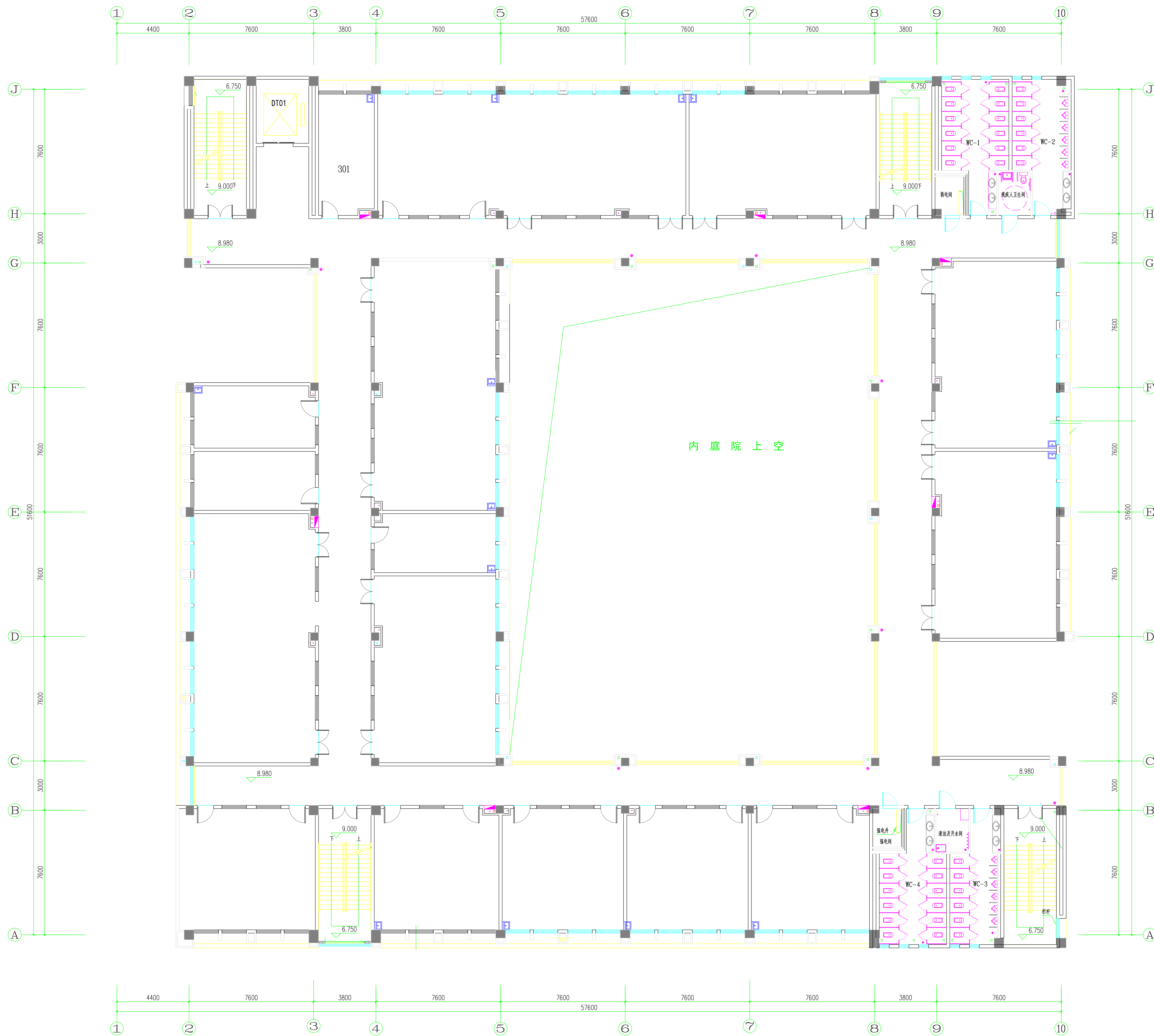
三层平面 1:100
