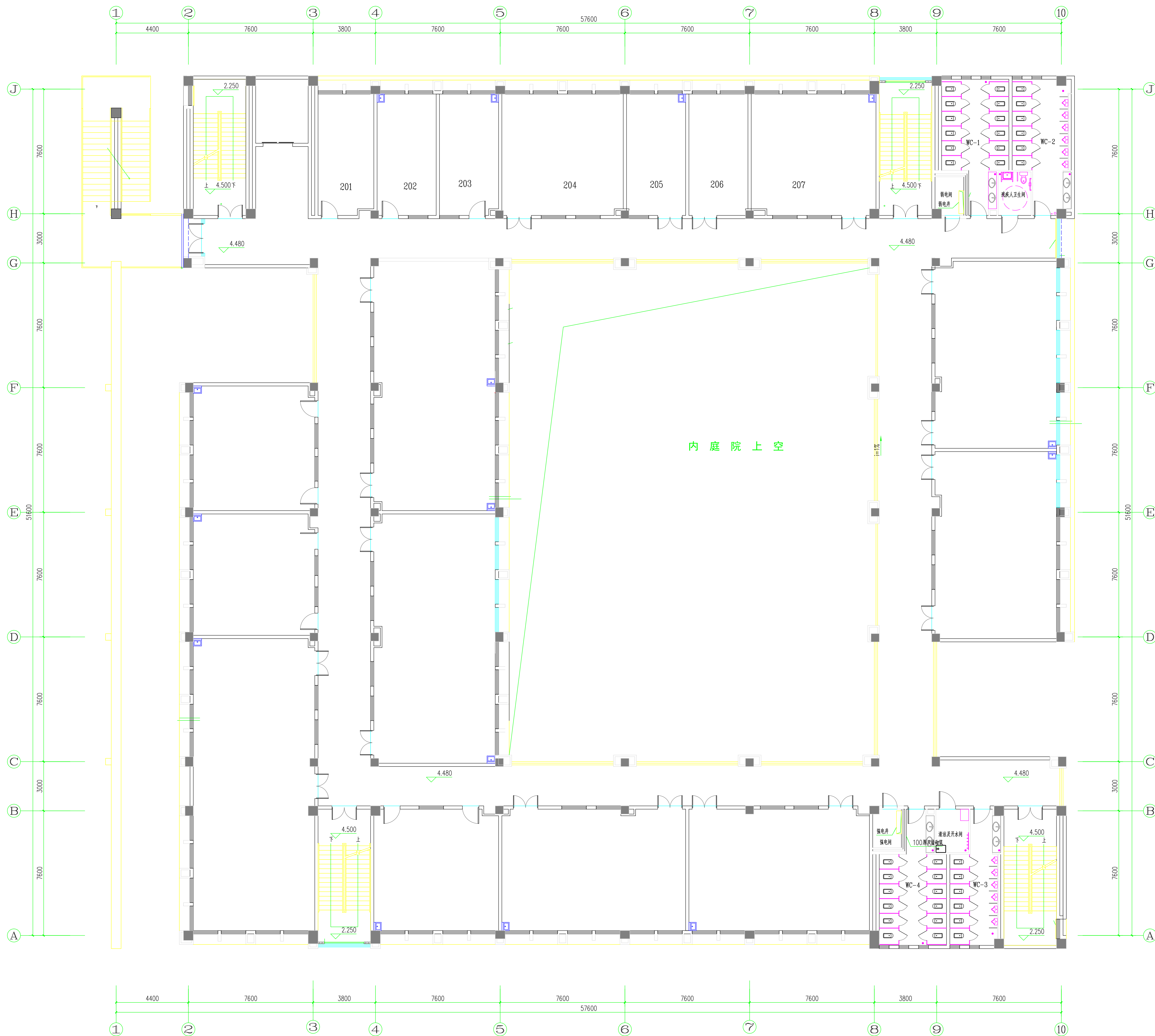
二层平面 1:100
